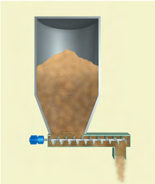
Bild 34: Silokonius mit waagerechter Räumschnecke (rechts: AZO GmbH + Co. KG)
