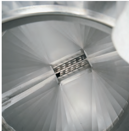
Bild 34: Silokonius mit waagerechter Räumschnecke (rechts: AZO GmbH + Co. KG)
