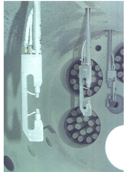
Abbildung 6: Messfühler für Staubkonzentrationsmessungen in einem pneumatisch befüllten Silo.
