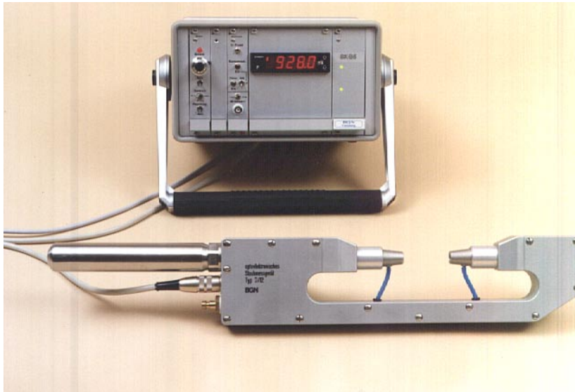
Abbildung 5: Direktanzeigendes Staubkonzentrationsmessgerät.
